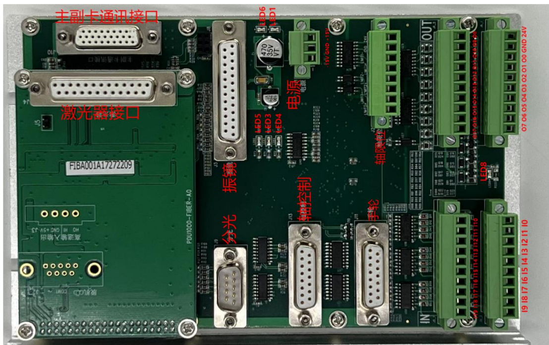
PCIE 端子板
